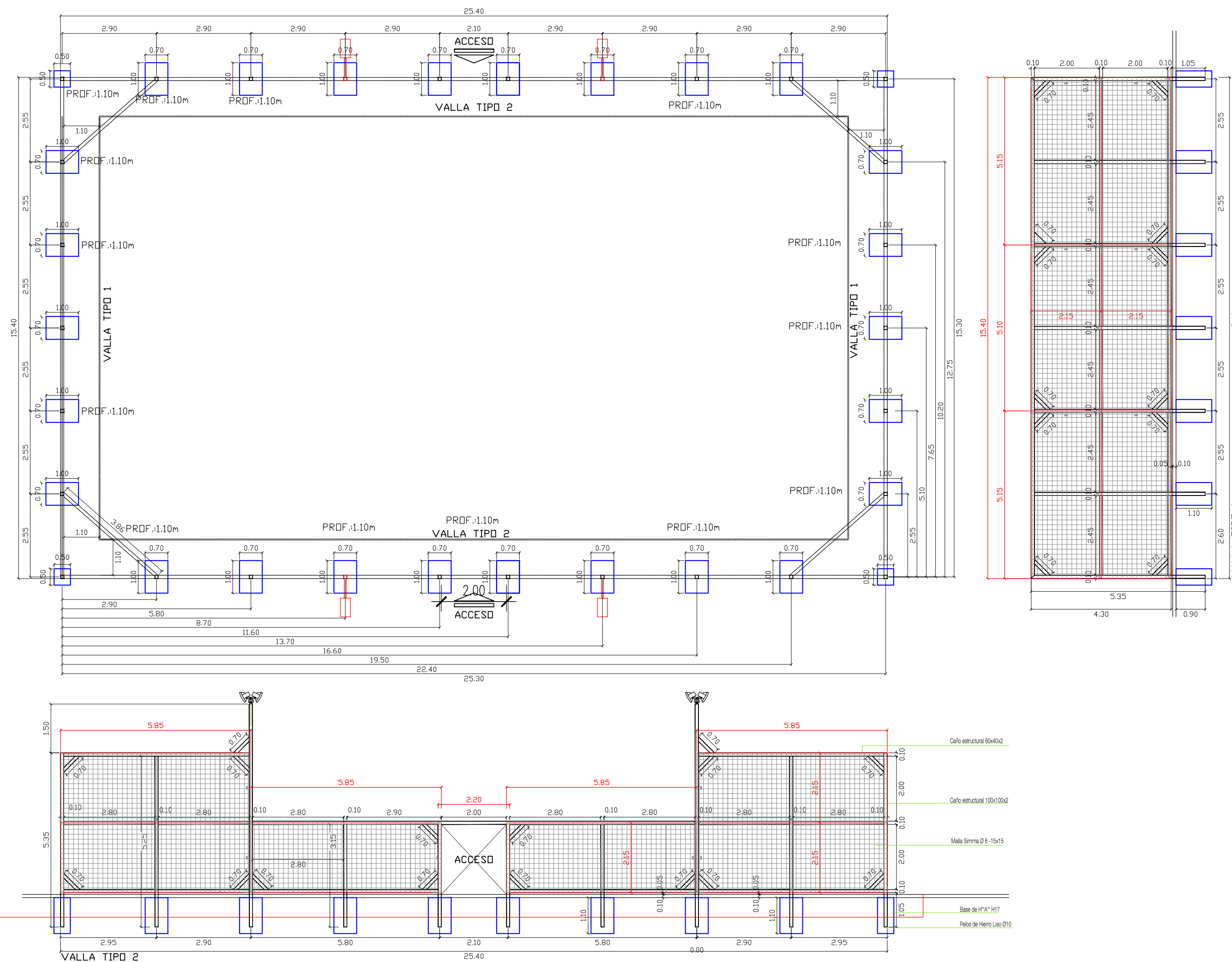
DETALLES VALLAS Esc. 1:100
